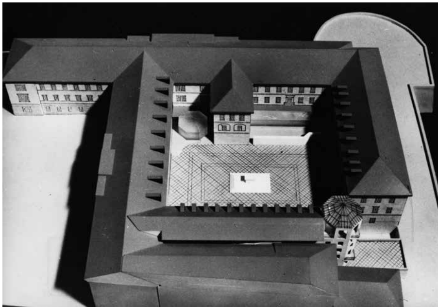
A keleti oldal felől készített felvételen jól látszik az aula bővítésének és a nagyterem előterének tervezett formája
