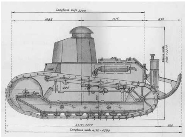
FIAT 3000/B harckocsi rajza (forrás: Istruzione sul carro armato mod. 1921 e mod. 1930. Rome, 1931. Tavola I.)
